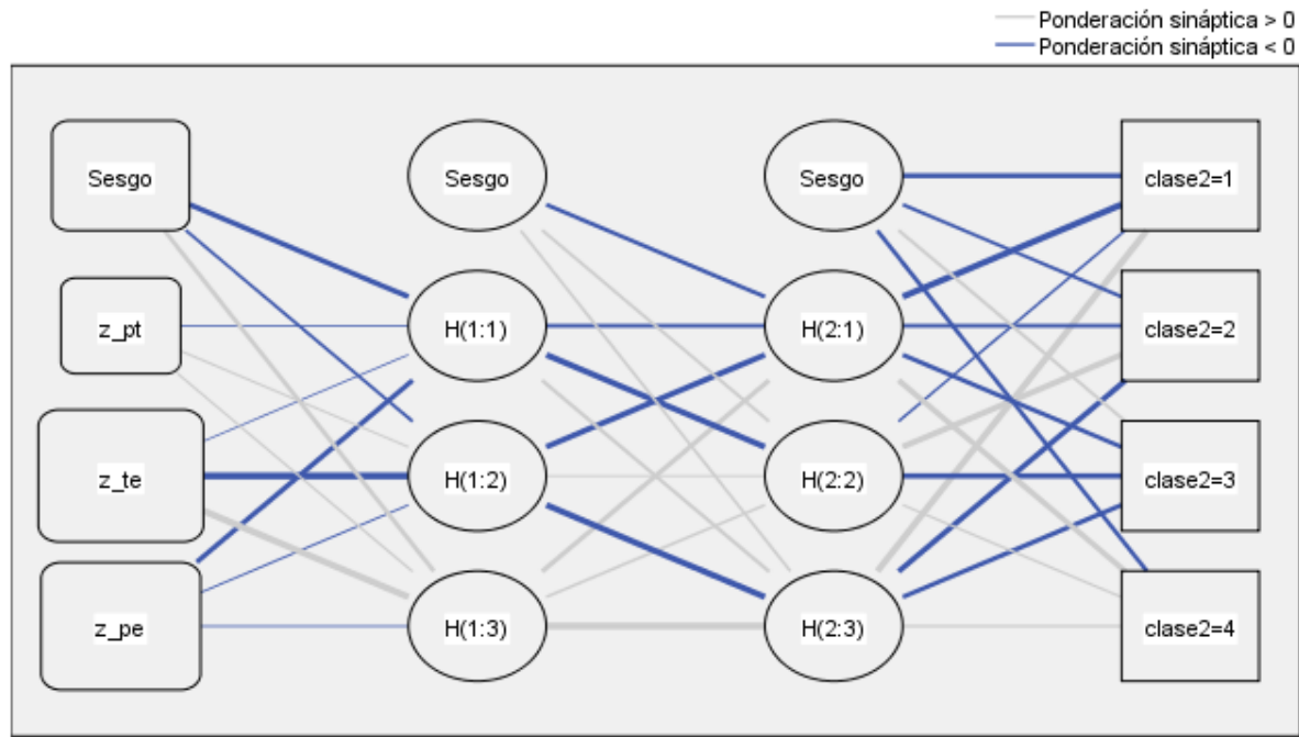
Figura 3.- Arquitectura de la red neuronal seleccionada.
